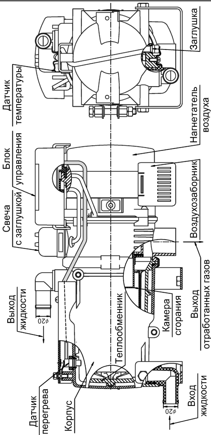
Рис. 4.3 – Основные узлы нагревателя
