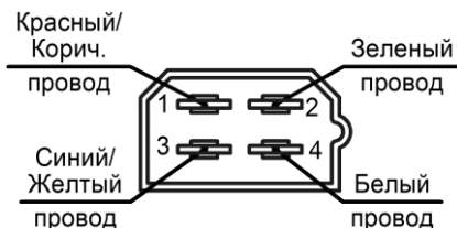
Рис. 6.1 – Установка контактов в колодку
