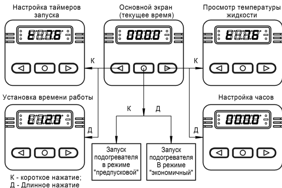
Рис. 6.3 – Алгоритм работы пульта.
