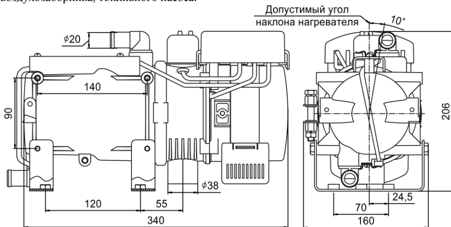
Рис. 7- Допустимые рабочие положения нагревателя
