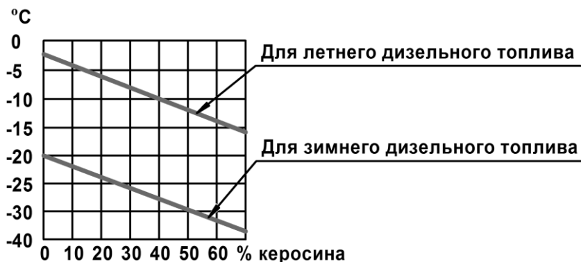
Рис. 12- Содержание керосина в смеси с дизельным топливом в зависимости от температуры окружающего воздуха
