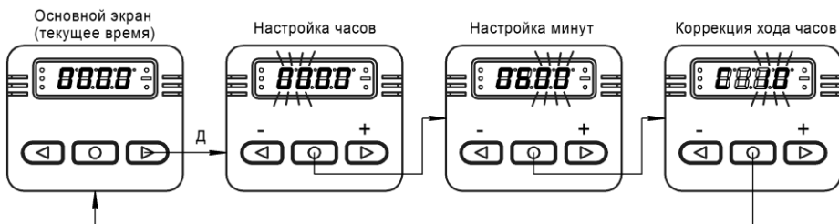
Рис. 6.4 – Настройка часов.
