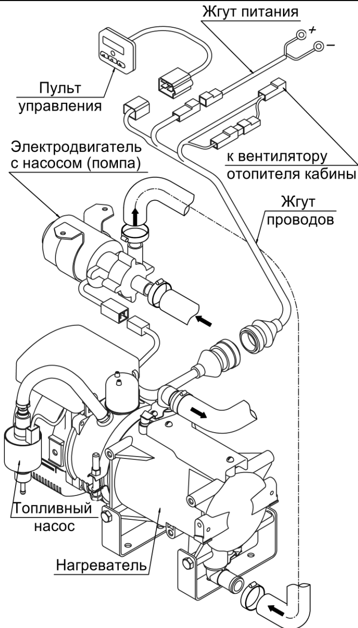
Рис. 4.2 – Основные узлы подогревателя.
