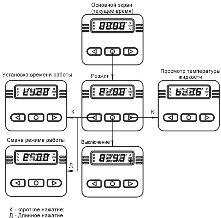
Рис.6.7 – Запуск подогревателя в режиме «предпусковой»
